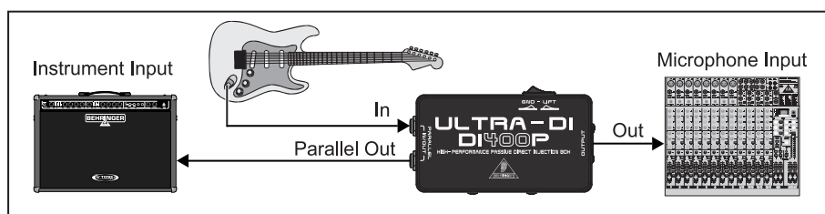
图 2：吉他 → 直接注入盒 → 吉他功放 / 调音台
