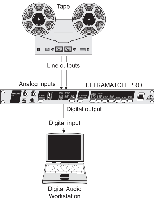
图 3.2: 例: 磁带录音的 A/D 转换
