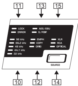
图 2.3: 输入区控制元件
