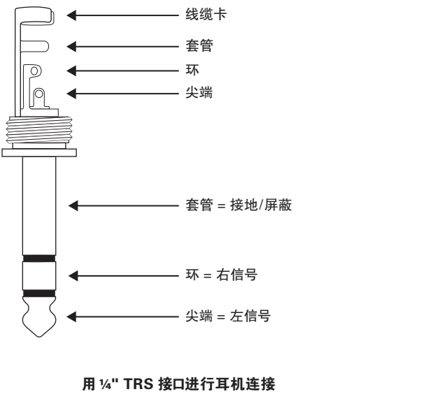
图 5.8: 耳机连接的正确连线配置
