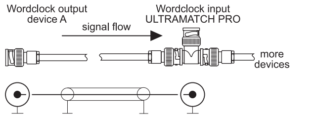
图 5.7: 字时钟输入的非平衡连接 (回路通过)
