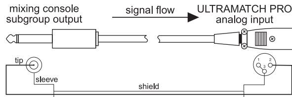
图 5.1: ULTRAMATCH PRO 非平衡输入
