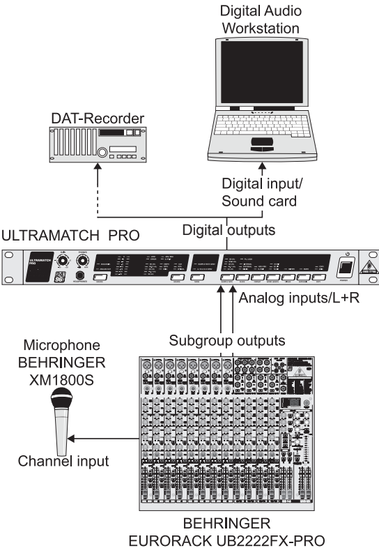
图 3.1: 例: 话筒信号 A/D 转换
