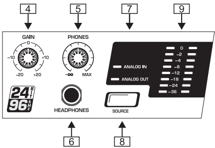
图 2.2: 输入区控制元件
