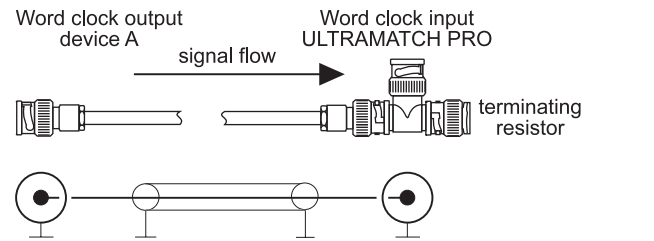
图 5.6: 非平衡连接 (终端) ULTRAMATCH PRO 的字时钟输入
