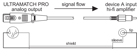
图 5.2: ULTRAMATCH PRO 非平衡输出
