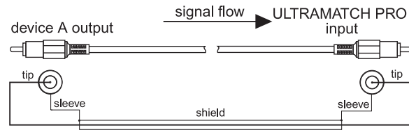
图 5.4: 在非平衡结构中连接 ULTRAMATCH PRO
