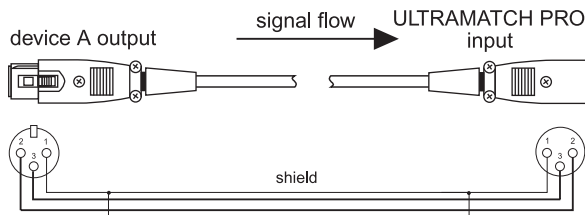
图 5.3: 在平衡结构中连接 ULTRAMATCH PRO
